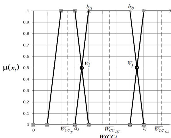
Рис. 1. Функція належності \mu(PV^{\varphi}_{N.i.j}) ЛЗ "СС"
