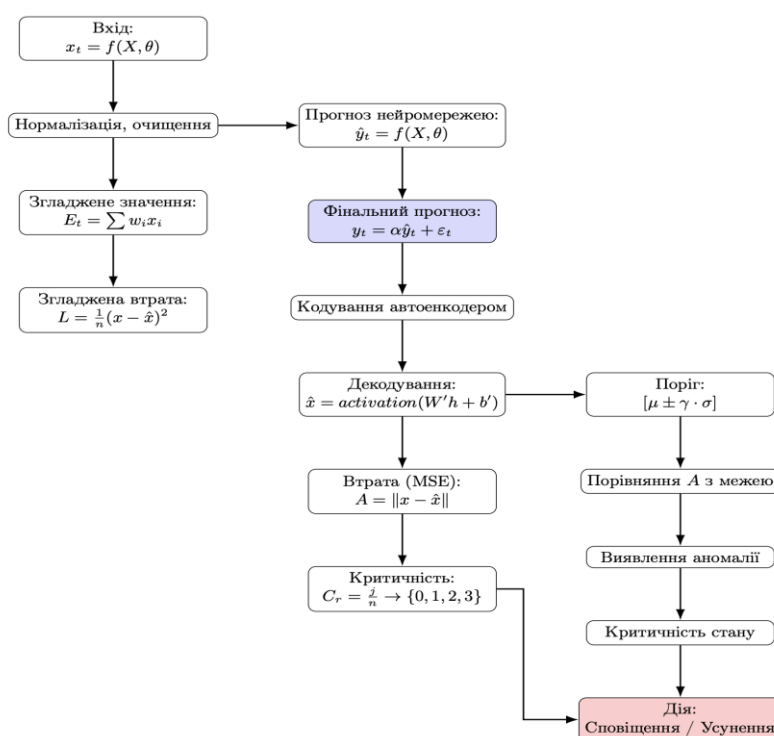
Рис. 1. Інтегрована модель прогнозування та виявлення аномалій
