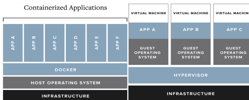
Рис. 6. Таблиця контейнерів, які спільно використовують системне ядро ОС машини, на відміну від віртуальних машин
