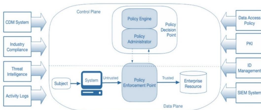
Рис. 1. Основні логічні компоненти архітектури нульової довіри
