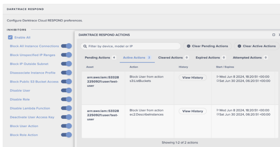
Рис. 4. Вбудована в платформу автономна відповідь, яка нейтралізує зловмисну активність
