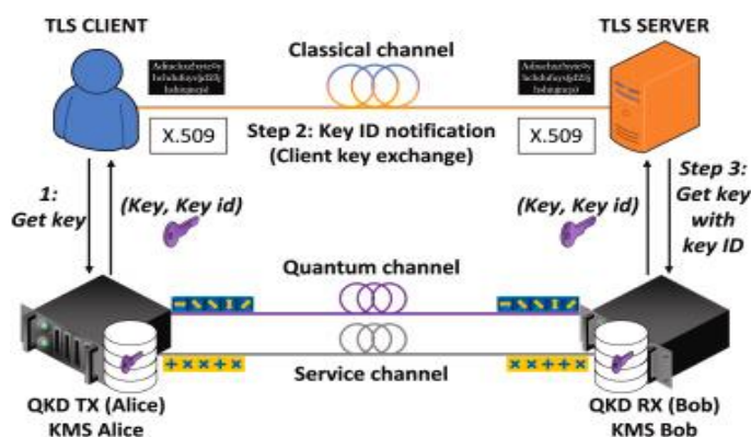
Рис. 9. Рівняння інтеграції QKD (квантового розподілу ключів) у класичні протоколи мережевої безпеки
